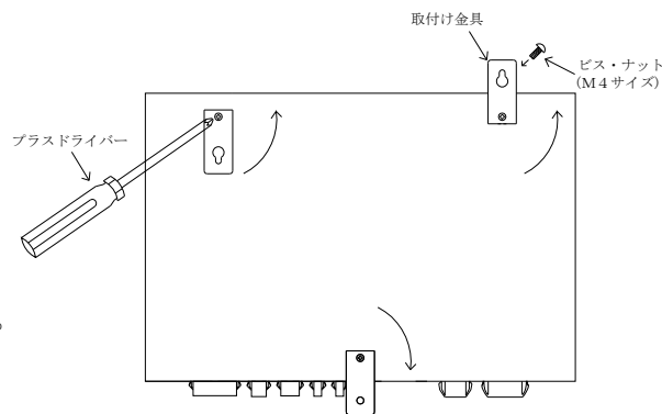
(BD2-K*****背面図)
