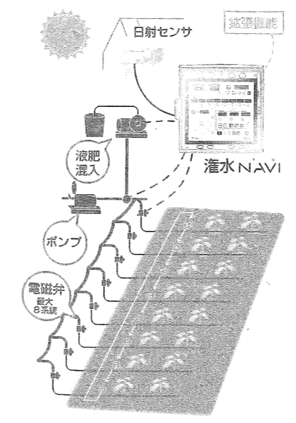
「灌水ナビ」構成図
